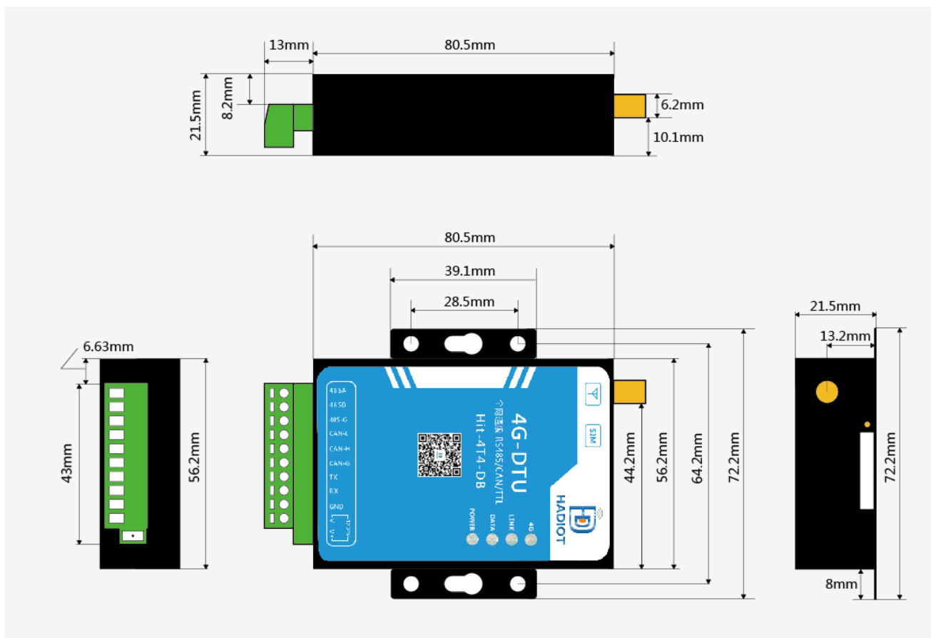
图 1 尺寸描述
