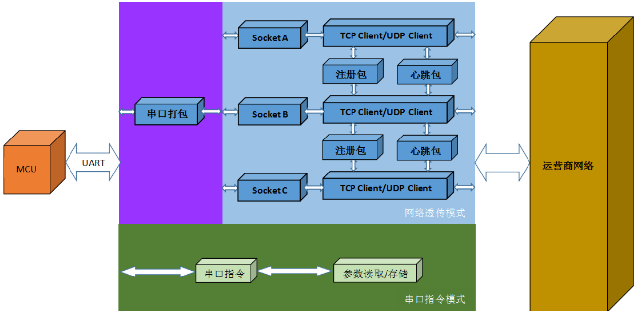
图 3 功能框图
