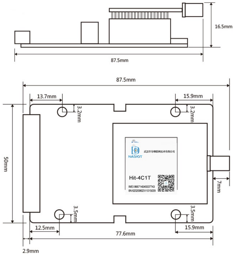
图 1 尺寸描述
